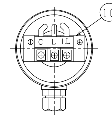
端子ボックス図
