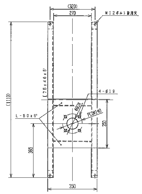
異型攪拌機架台正面図詳細
